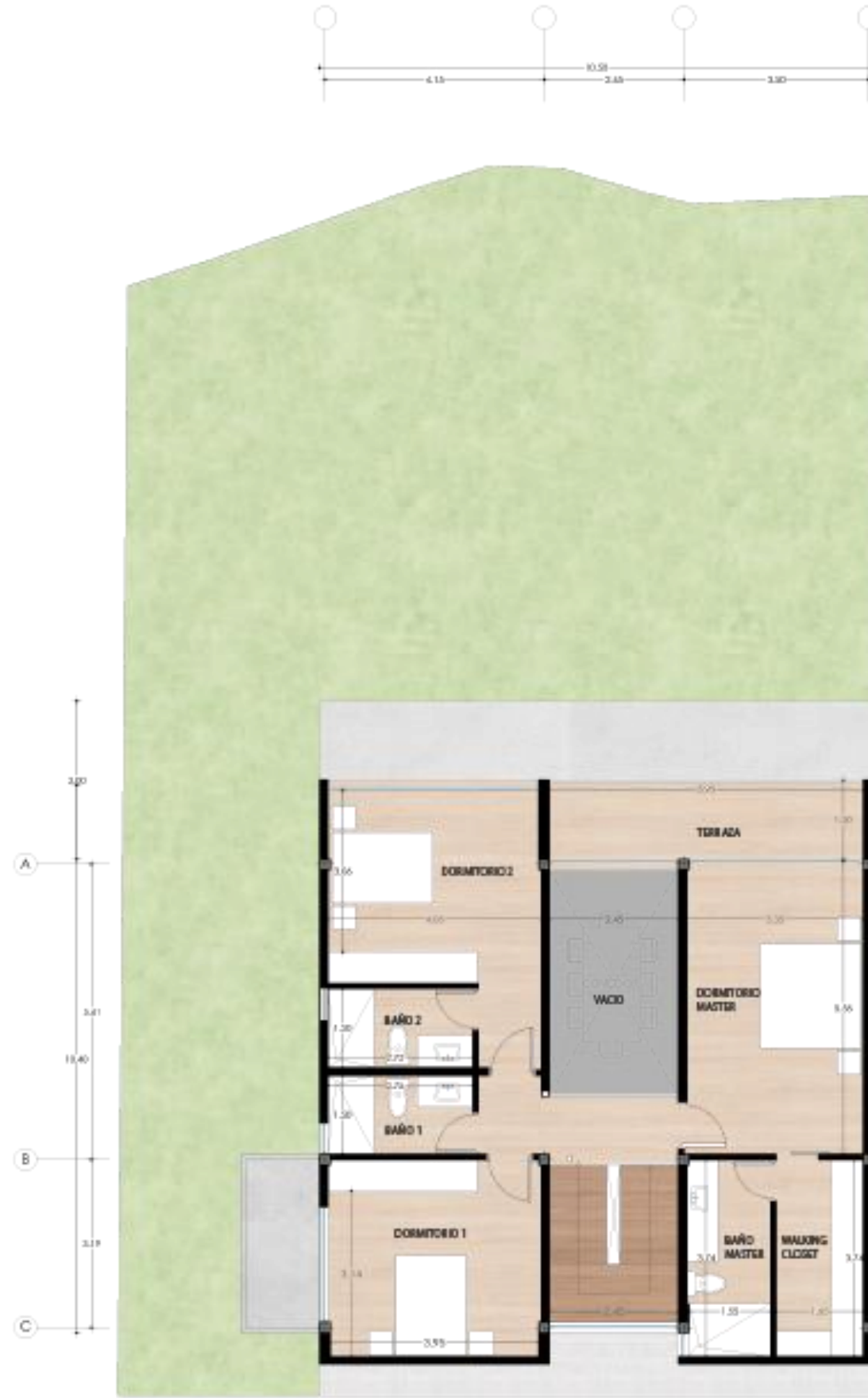
PLANTA ALTA CASA TIPO A AREA: 116,55m 2
