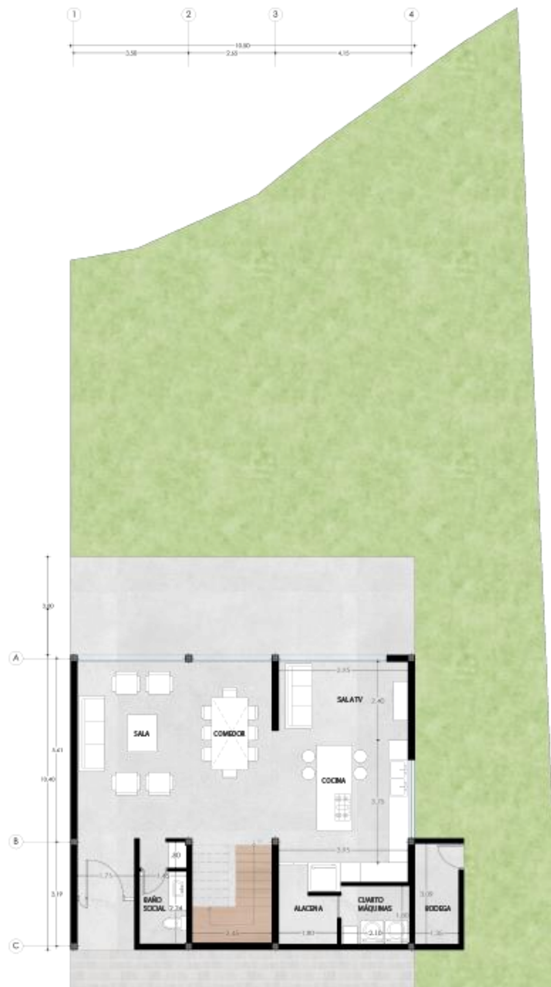
PLANTA BAJA CASA TIPO A AREA: 131,09m 2
