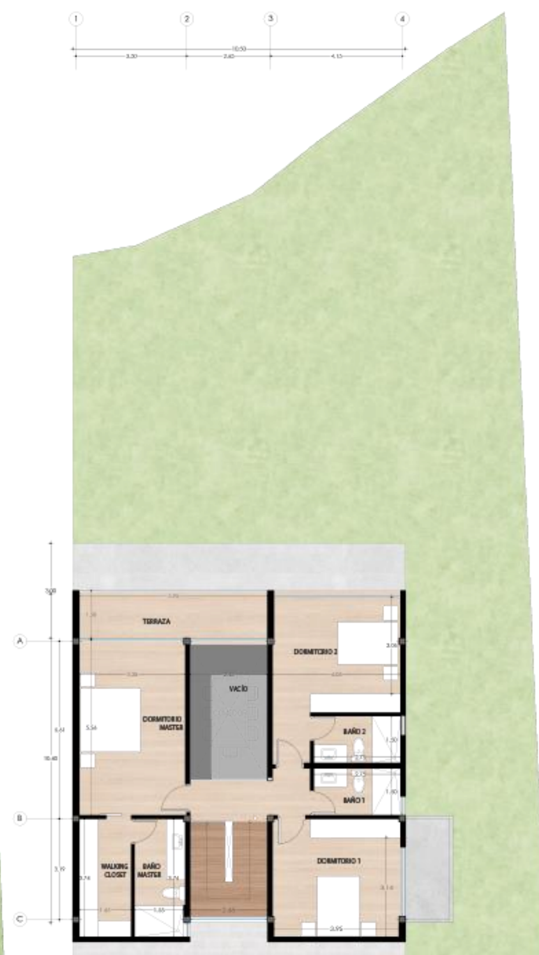
PLANTA ALTA CASA TIPO A AREA: 116,55m 2
