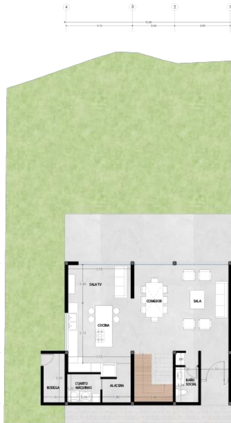
PLANTA BAJA CASA TIPO A AREA: 131,09m 2
