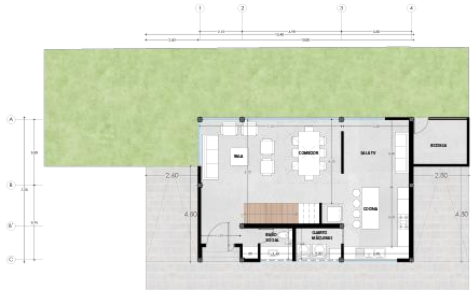
PLANTA BAJA CASA 5A AREA: 97,17m 2
